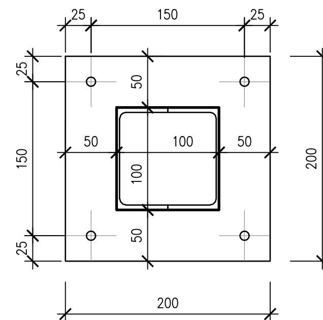
PATNÍ PLECH ⑥
