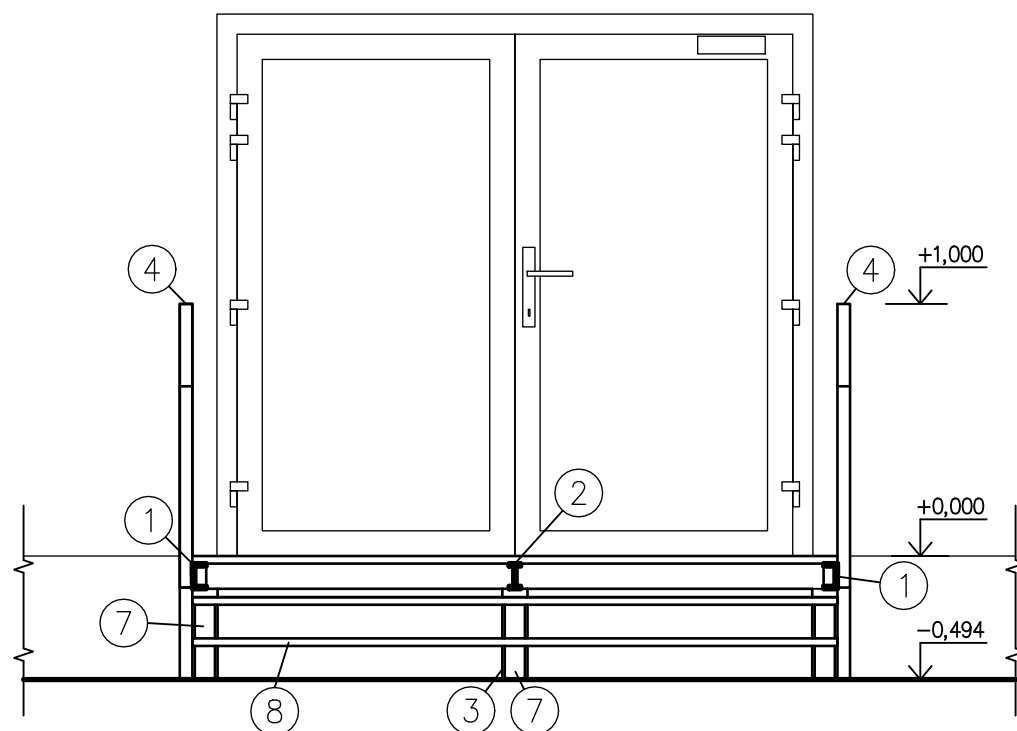
ČELNÍ POHLED
