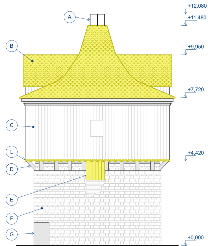
JIHOZÁPADNÍ POHLED
