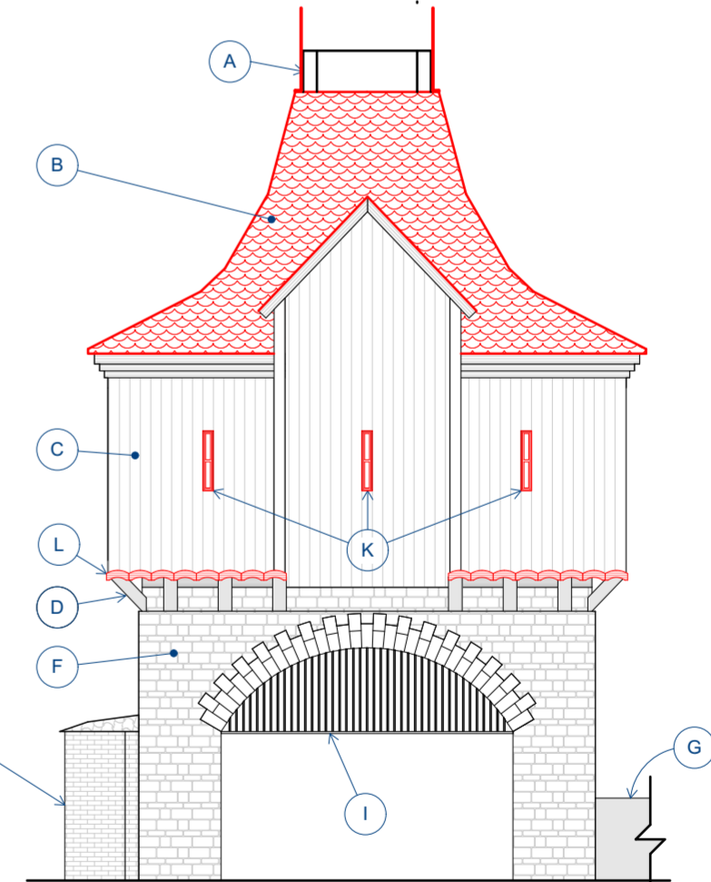
SEVEROZÁPADNÍ POHLED
