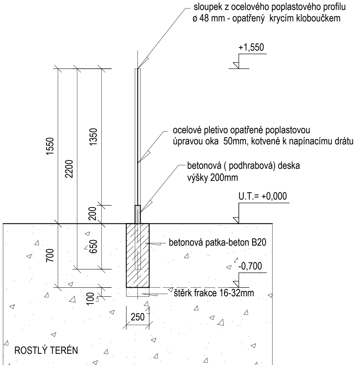
POVRCHOVÁ ÚPRAVA VÝPLNĚ OPLOCENÍ- OCELOVÉ POPLASTOVÉ PLETIVO
