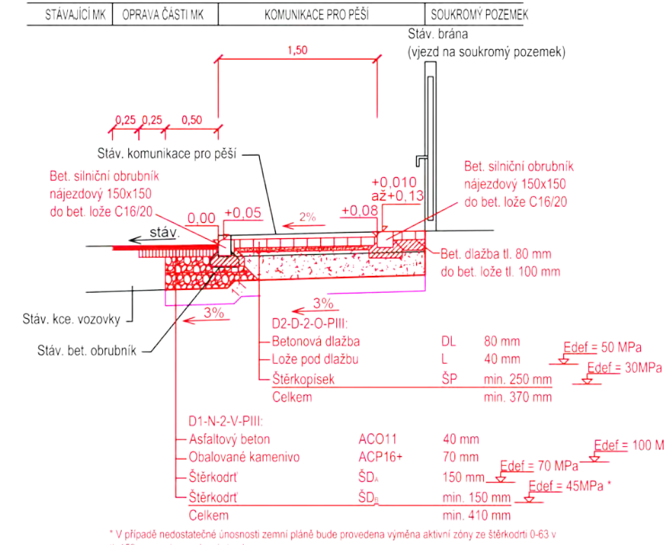
VZOROVÝ PŘÍČNÝ ŘEZ Č. 1 M 1:50
