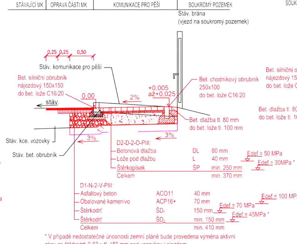
VZOROVÝ PŘÍČNÝ ŘEZ Č. 7 M 1:50
