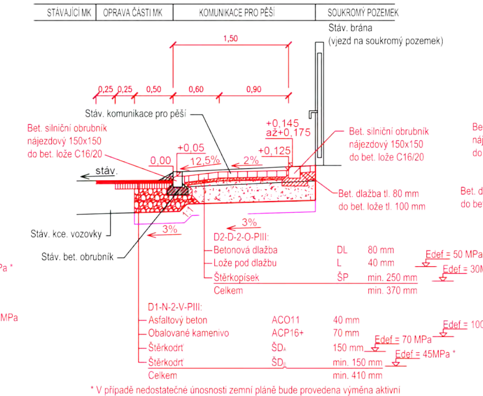
VZOROVÝ PŘÍČNÝ ŘEZ Č. 5 M 1:50
