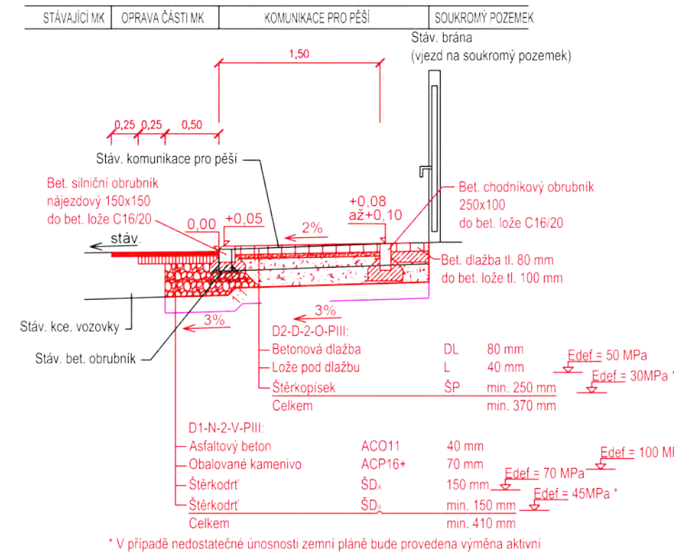
VZOROVÝ PŘÍČNÝ ŘEZ Č. 3 M 1:50
