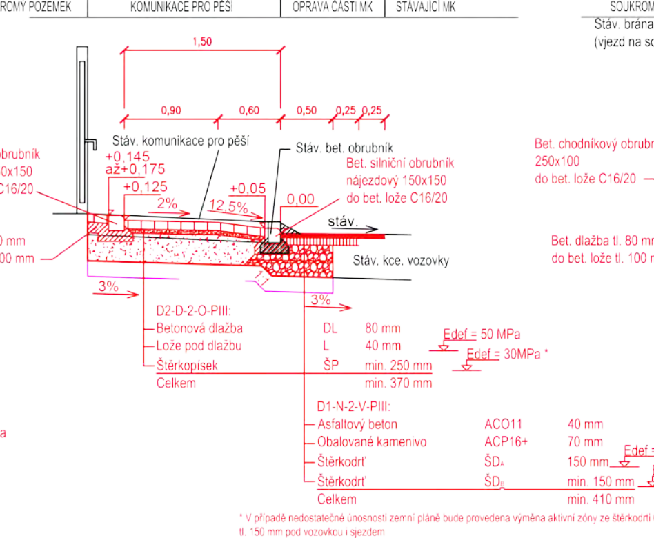
VZOROVÝ PŘÍČNÝ ŘEZ Č. 9 M 1:50
