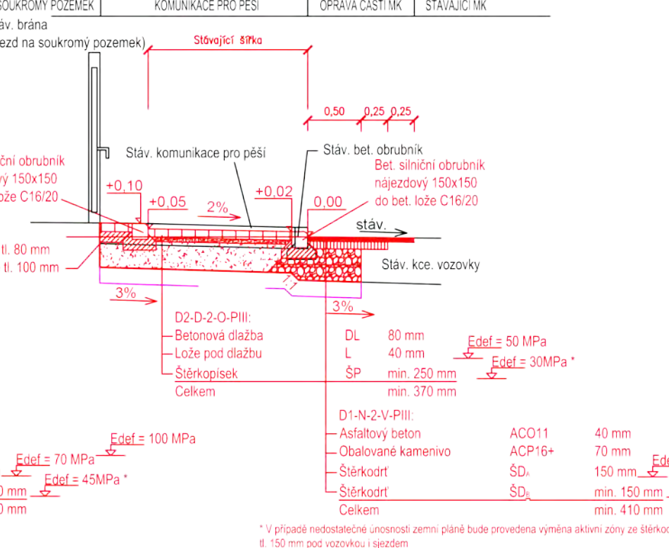
VZOROVÝ PŘÍČNÝ ŘEZ Č. 11 M 1:50
