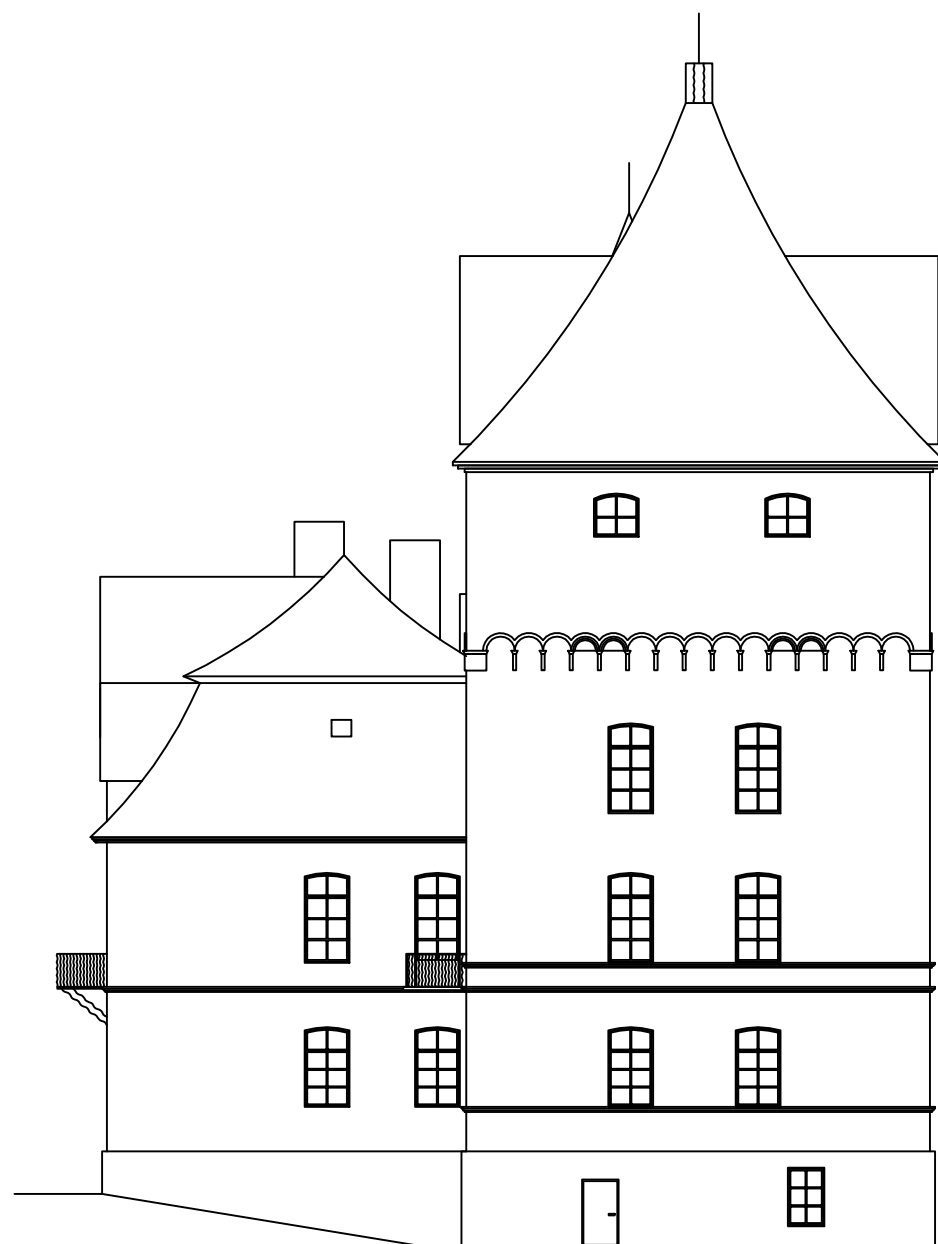
SEVEROVÝCHODNÍ POHLED
