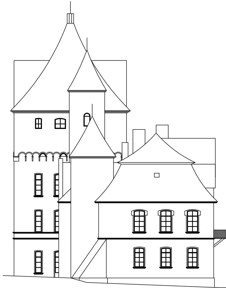
JIHOZÁPADNÍ POHLED
