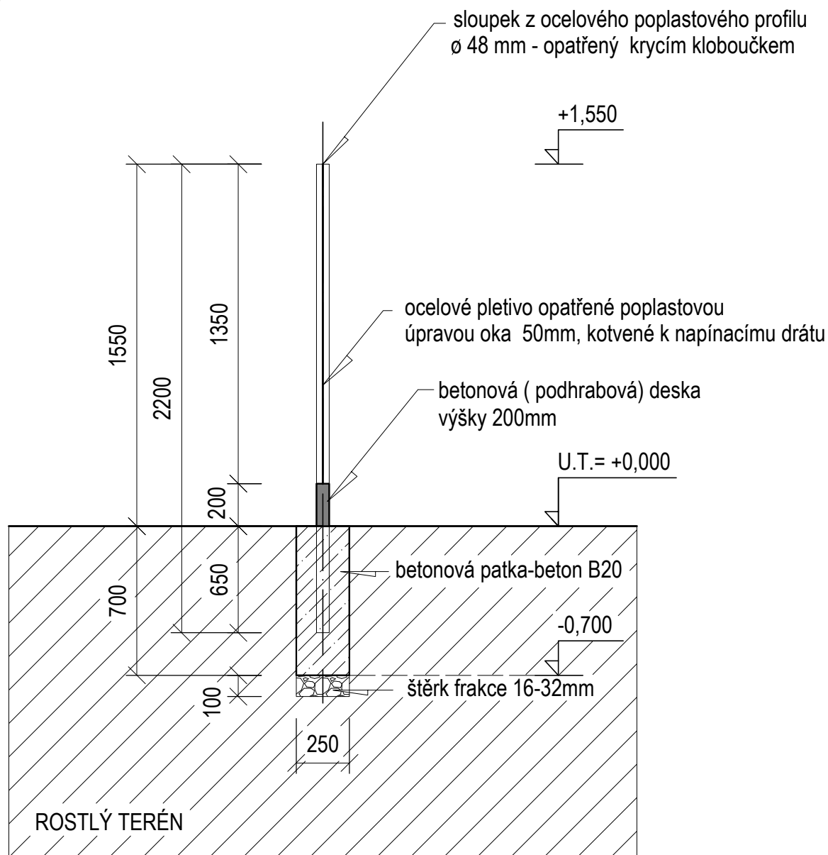
POVRCHOVÁ ÚPRAVA VÝPLNĚ OPLOCENÍ- OCELOVÉ POPLASTOVÉ PLETIVO
